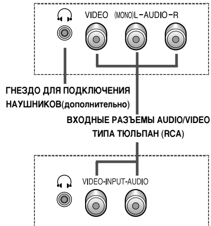
Передняя панель телевизора
