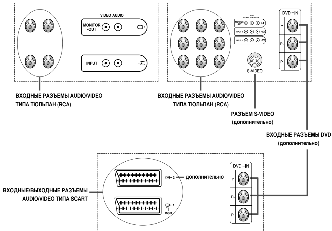
Задняя панель телевизора
