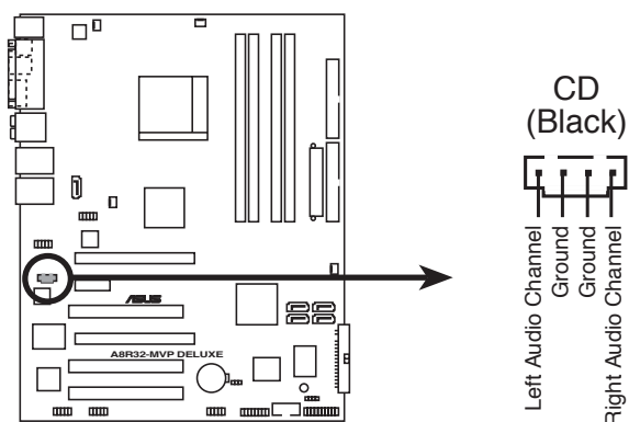
Connecteurs audio internes de l'A8R32-MVP DELUXE
