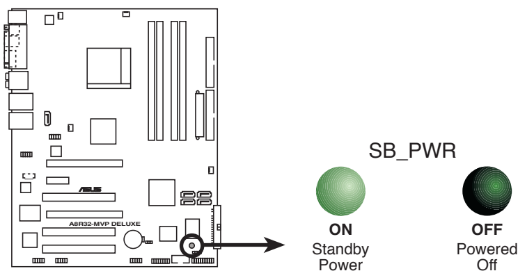
LED embarquée de l'A8R32-MVP DELUXE
