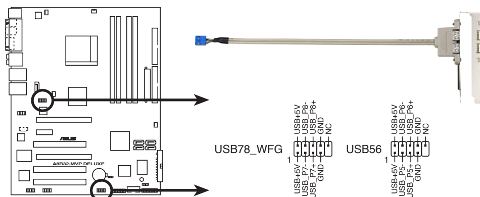
Connecteur USB 2.0 de l'A8R32-MVP DELUXE
