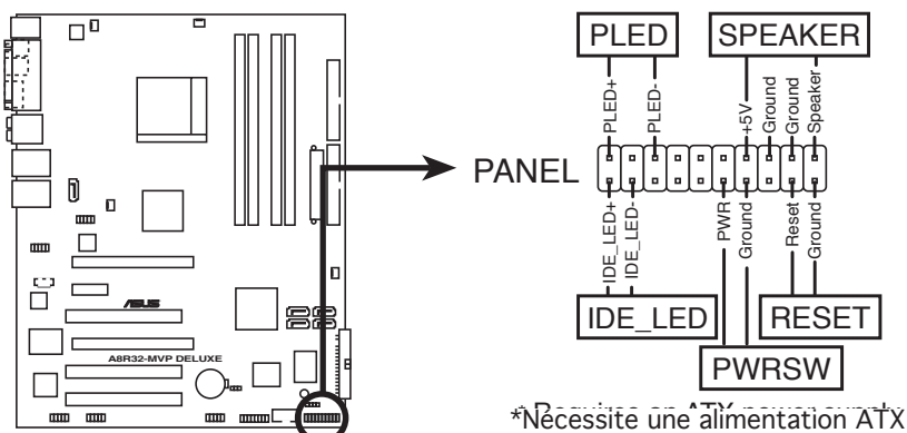
Connecteur System Panel de l'A8R32-MVP DELUXE
