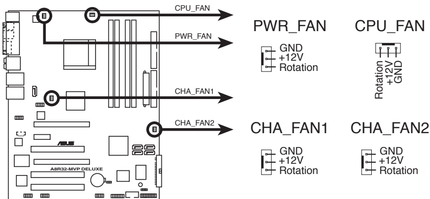
Connecteur ventilateurs de l'A8R32-MVP DELUXE
