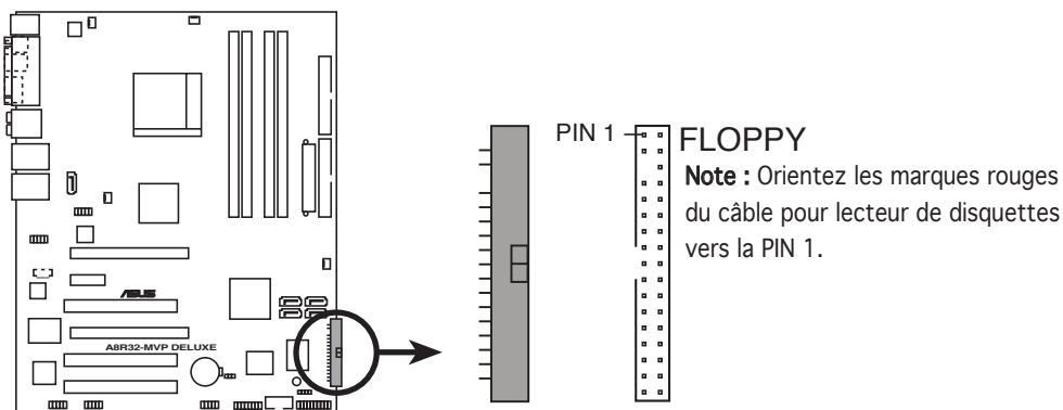
Connecteur lecteur de disquettes de l'A8R32-MVP DELUXE
