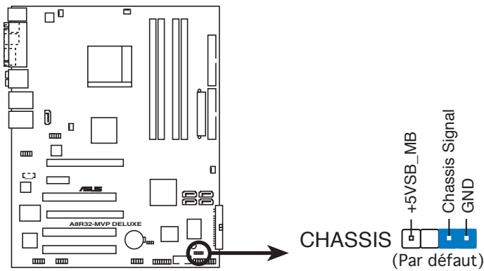
Connecteur Châssis intrusion de l'A8R32-MVP DELUXE
