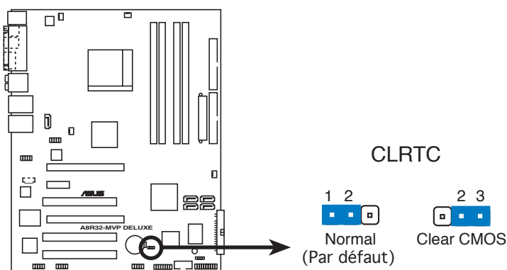
Clear RTC RAM de l'A8R32-MVP DELUXE
