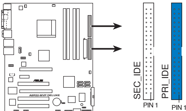
Connecteurs IDE de l'A8R32-MVP DELUXE
