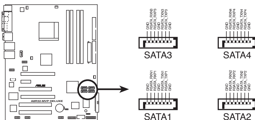
Connecteurs SATA de l'A8R32-MVP DELUXE
