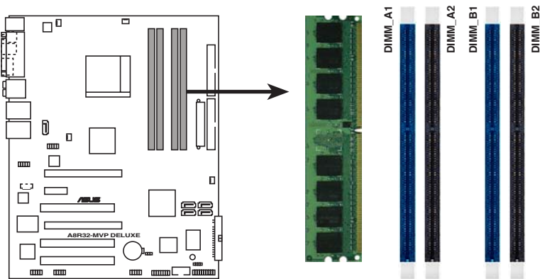
Sockets 184 broches DIMM DDR de l'A8R32-MVP DELUXE
