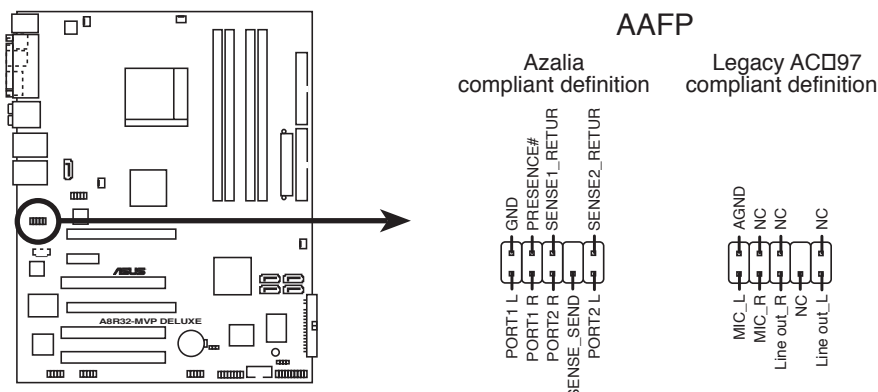
Connecteur Front panel audio de l'A8R32-MVP DELUXE
