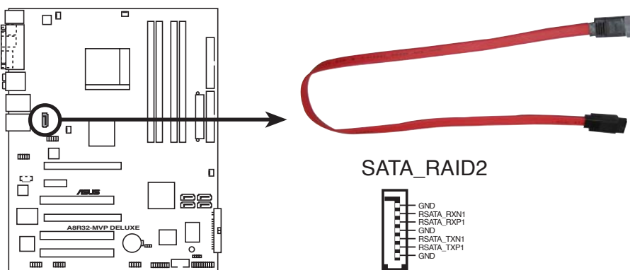
Connecteurs RAID SATA de l'A8R32-MVP DELUXE
