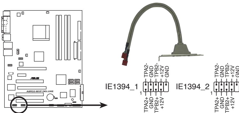
Connecteur IEEE 1394 de l'A8R32-MVP DELUXE
