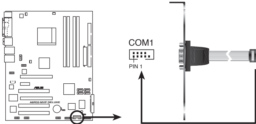
Connecteur port COM de l'A8R32-MVP DELUXE
