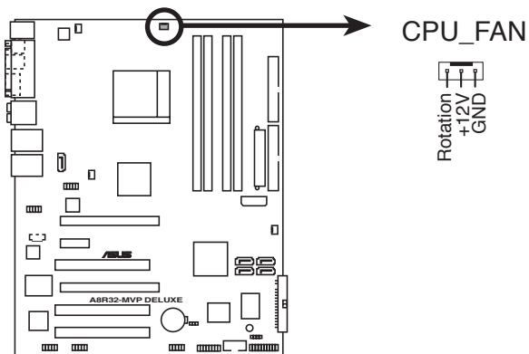
Connecteur du ventilateur CPU de l'A8R32-MVP DELUXE
